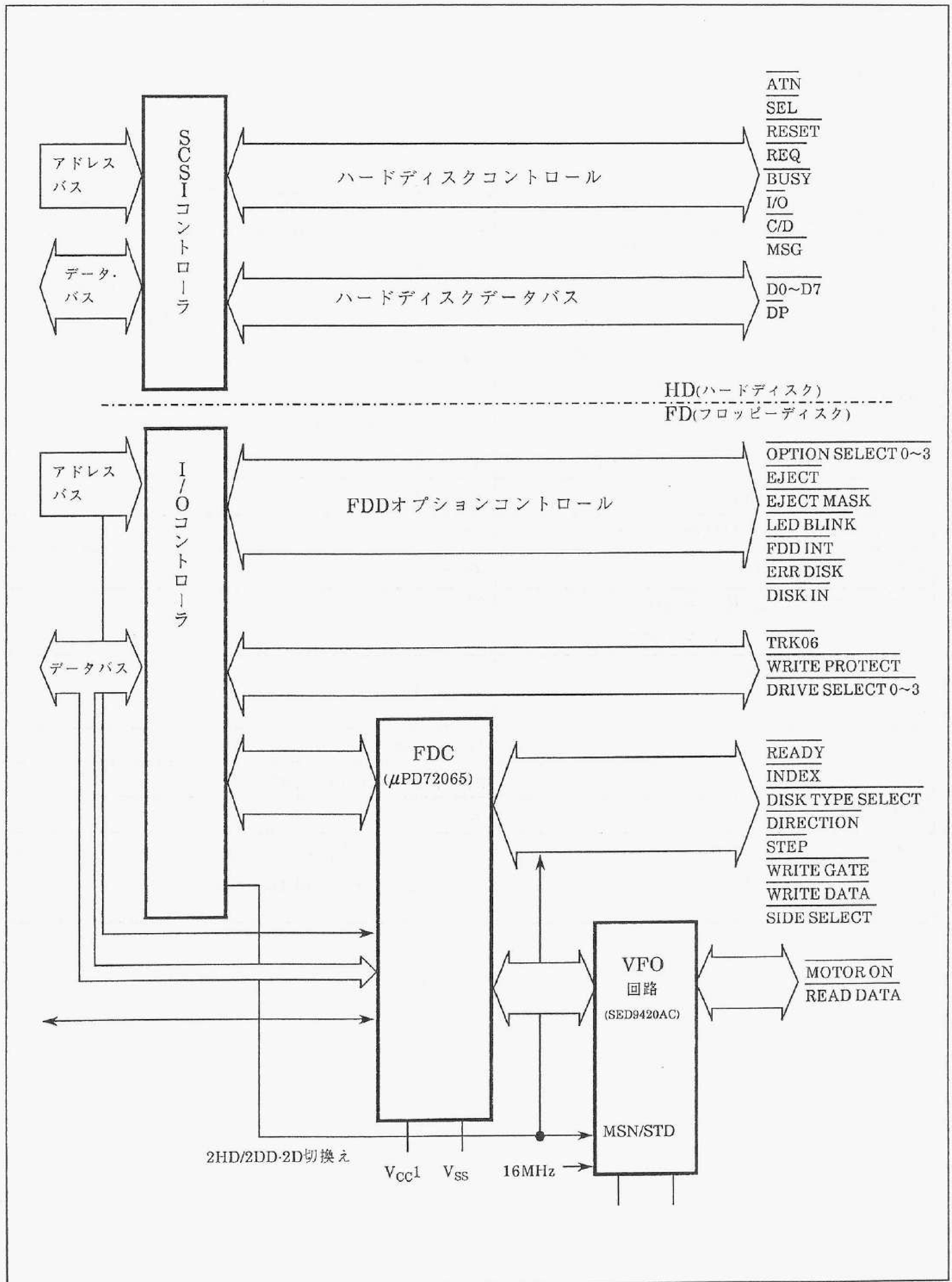
図9-1 FDD/HDD周辺ブロック図
