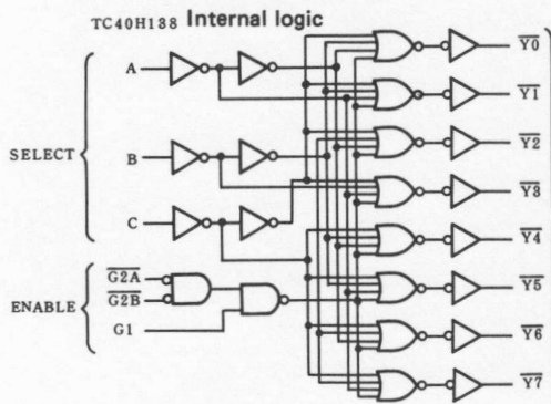
Truth Table
